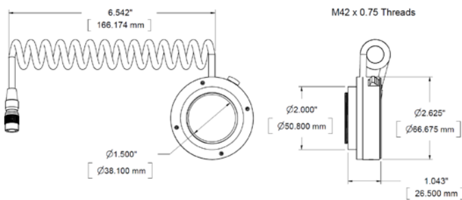
LC-2A-T EF-M42x0.75 Lens Adapter
